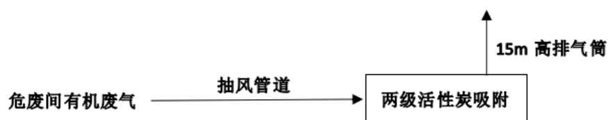
图 3.1 危险废物暂存间废气处理工艺流程图
