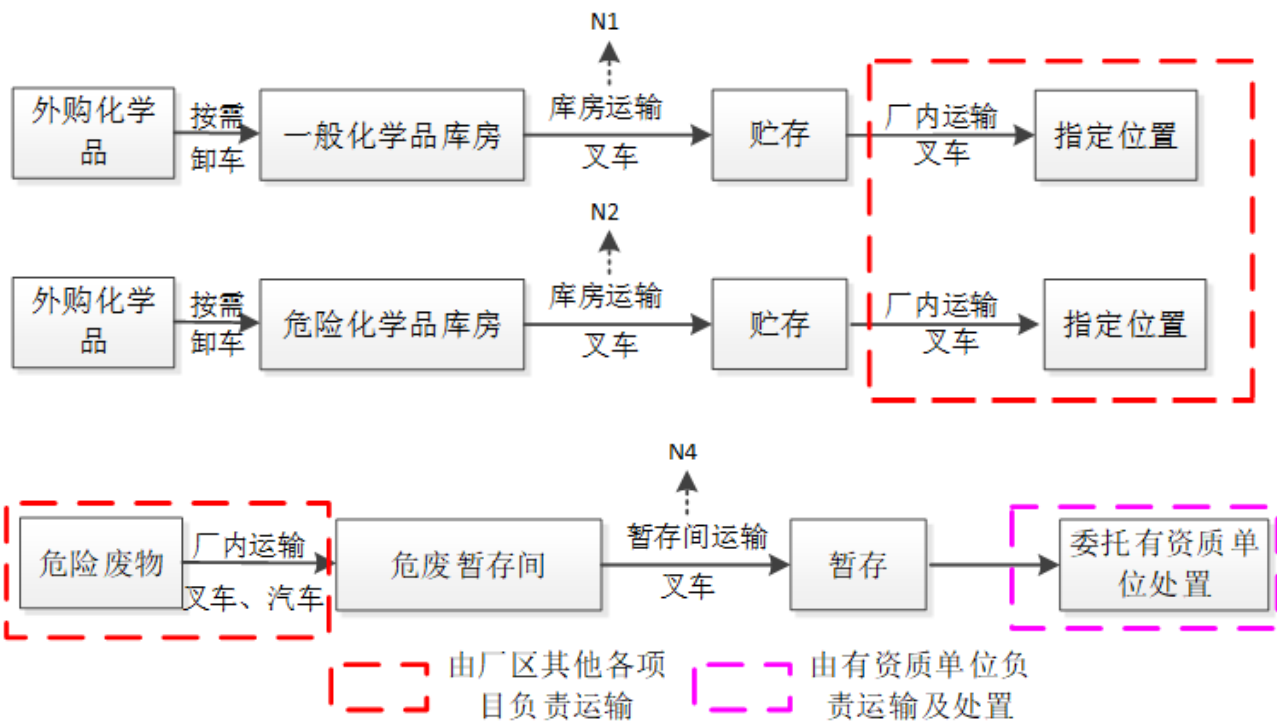
图 2.3 建设项目一阶段工艺流程及产污环节图
