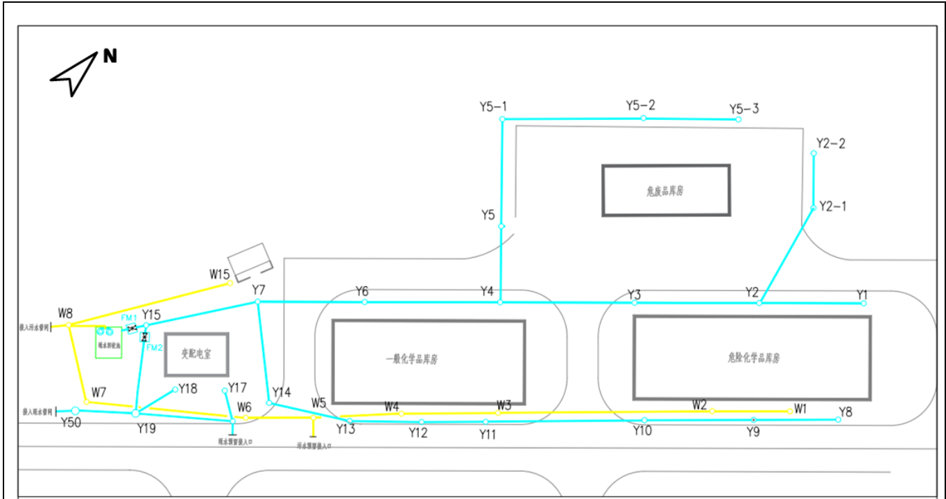
图 2.2 建设项目一阶段总平面布置图
